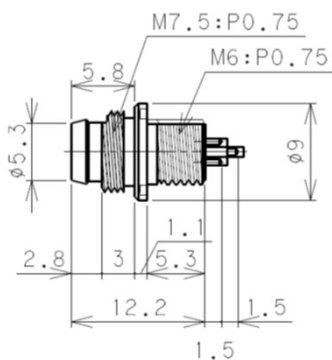
<オスレセプタクル/後止タイプ> <ネジロック方式>
