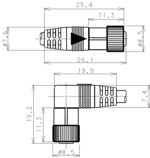
<メスプラグ/ネジロック方式>
